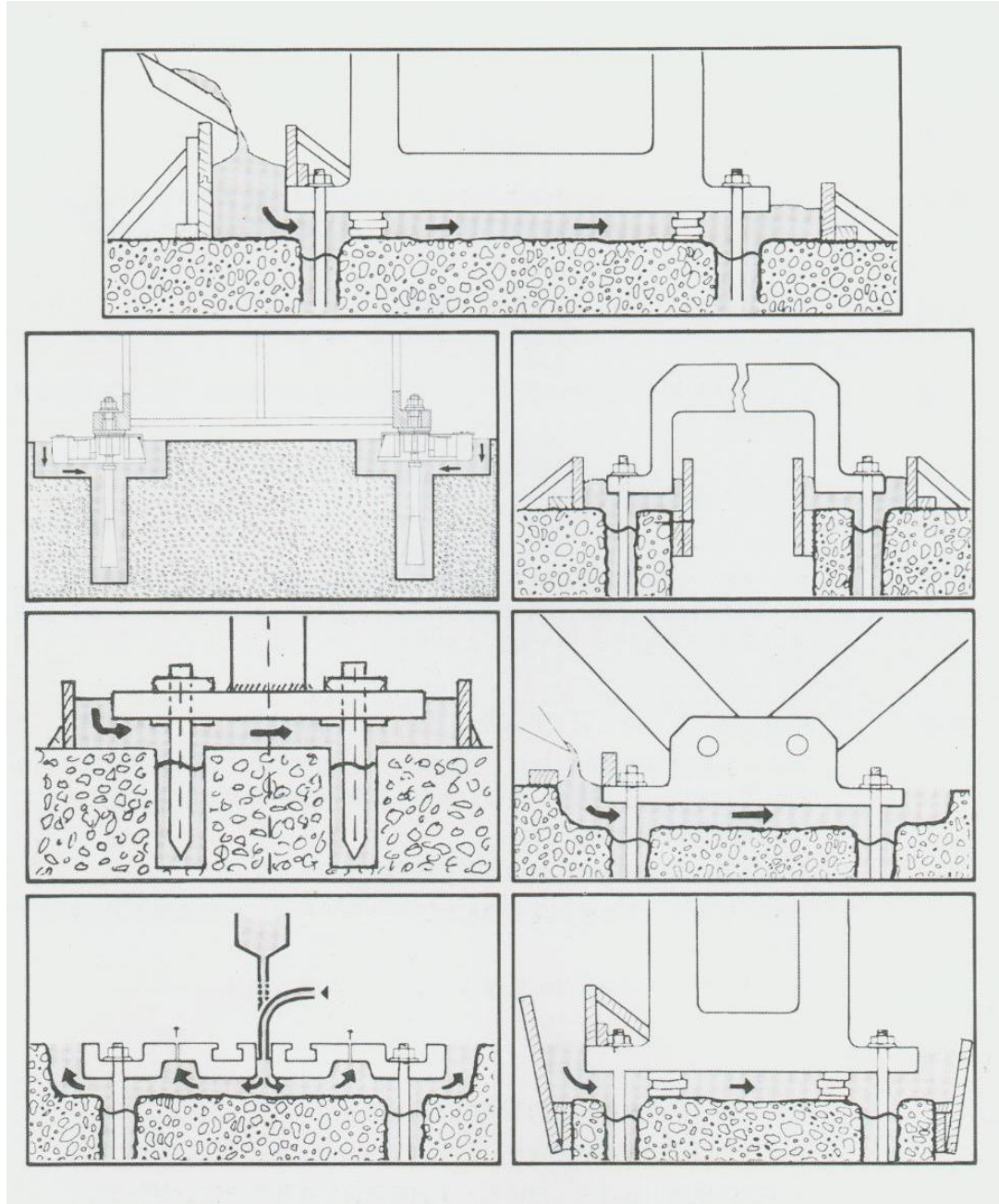
Hình ảnh minh họa thi công vữa tự chảy không co VICTA-GROUT
